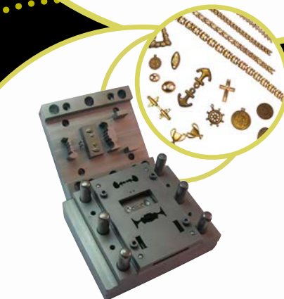
STAMPI E TRANCE PER VARI ELEMENTI MODULS FOR VARIOUS ELEMENTS
